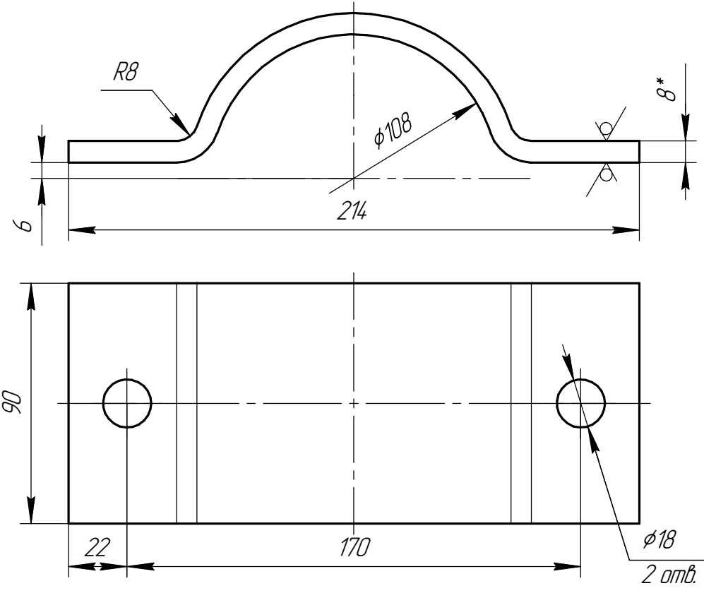
Дет. поз. 2 (1:2)
